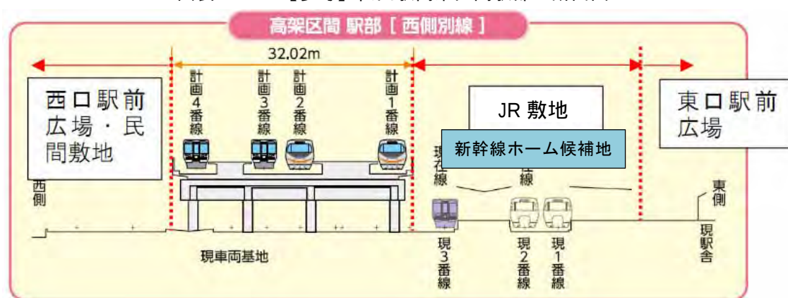
図表 2-13 【参考】松山駅高架区間駅部の断面図
